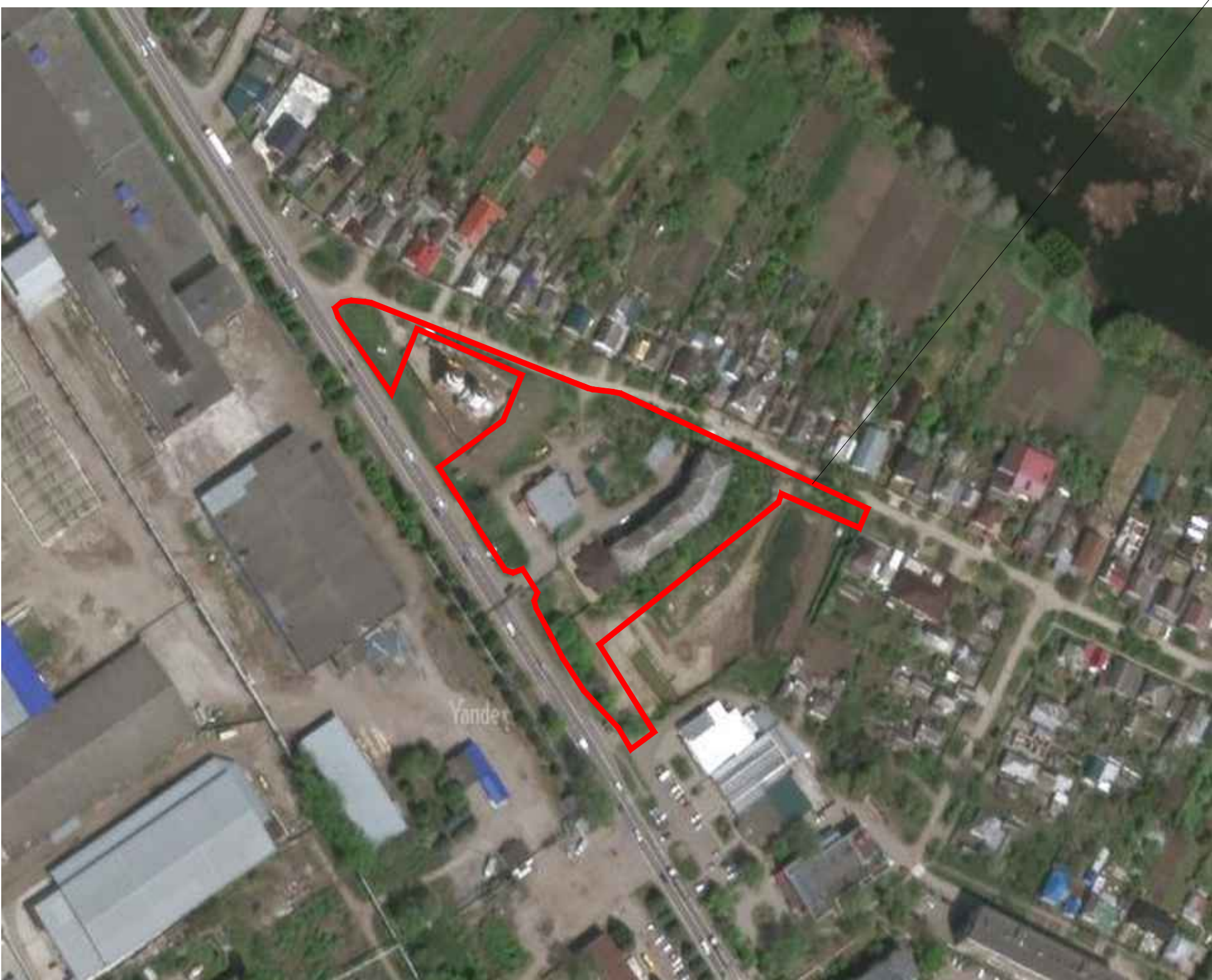
ПРОЕКТИРУЕМЫЙ УЧАСТОК
