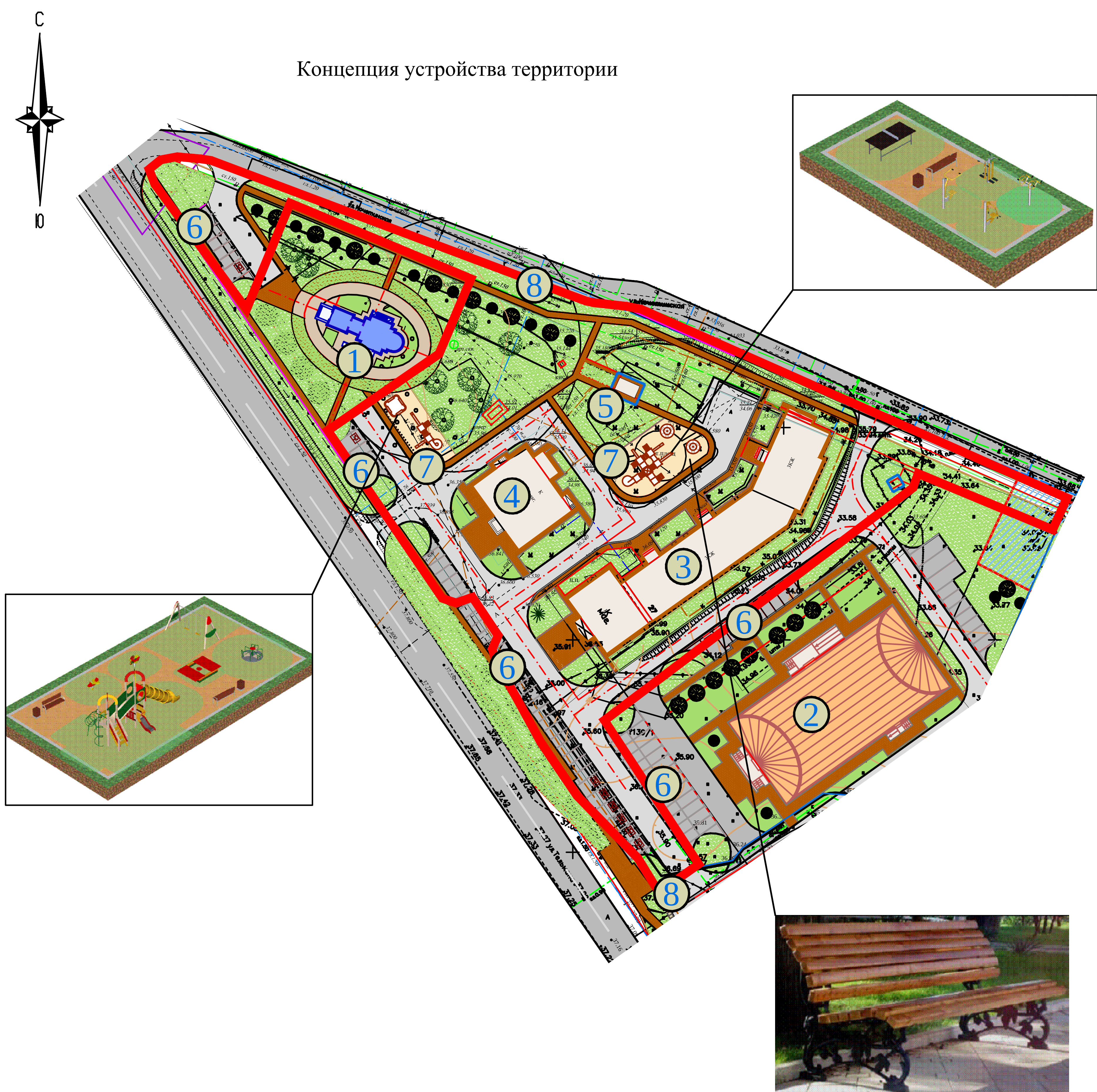
ПРОЕКТИРУЕМЫЙ УЧАСТОК
